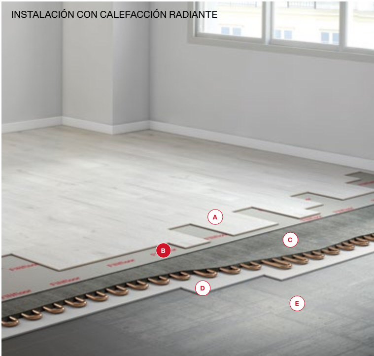
A FINFLOOR B MANTA SILENT ELITE FINFLOOR C CALEFACCIÓN RADIANTE D AISLANTE E SOLERA
